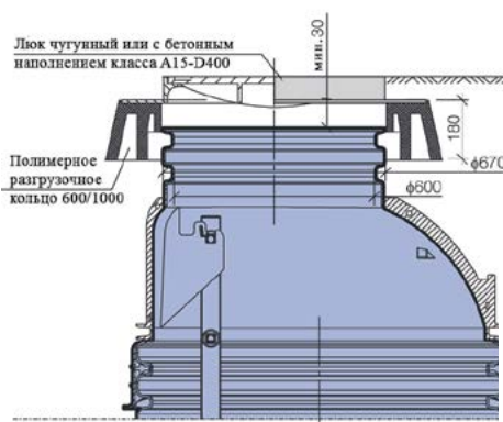
Люк A15, B125 или D400 на полимерном разгрузочном кольце
