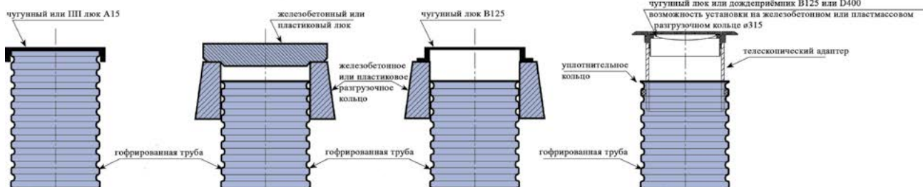
Люк A15 на гофрированной трубе
